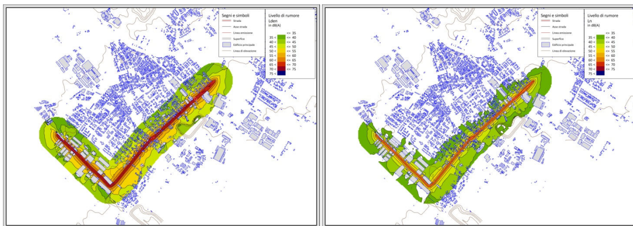
Figura 7 Mappe acustiche per i livelli L_{den} (a sinistra) e L_{night} (a destra) per il dominio di simulazione attorno al tratto di S.P. 109 di competenza del Comune di Nerviano
