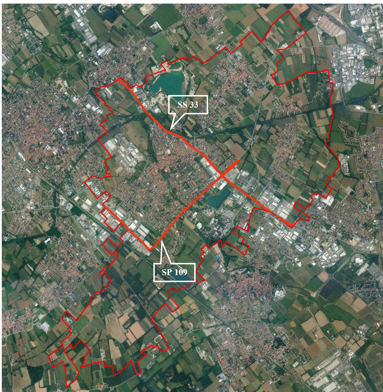
Figura 1 Perimetrazione del Comune di Nerviano con indicazione dei tratti stradali di sua competenza da sottoporre a mappatura acustica
