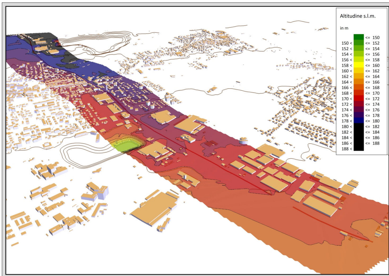
Figura 4 Discretizzazione del dominio di simulazione attorno al tratto di S.S. 33 del Sempione di competenza del Comune di Nerviano
