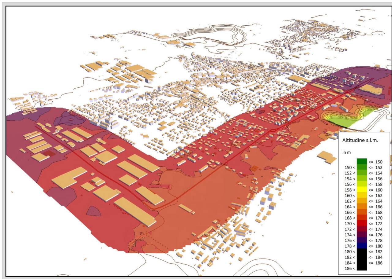
Figura 5 Discretizzazione del dominio di simulazione attorno al tratto di S.P. 109 di competenza del Comune di Nerviano
